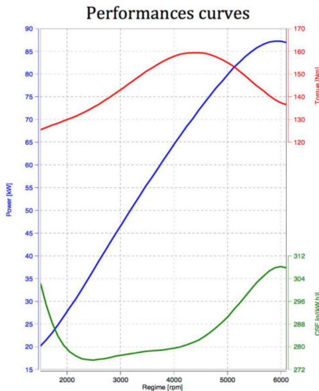
Relation couple / puissance moteur 1,6 VTI inj indirecte 88 kW 120 ch PSA
